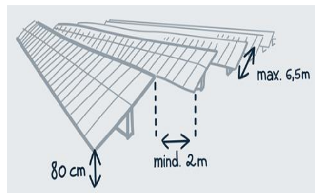
Abbildung 1: Beispiel Abmessung einer naturverträglichen PV, Bild: Photovoltaic Austria
